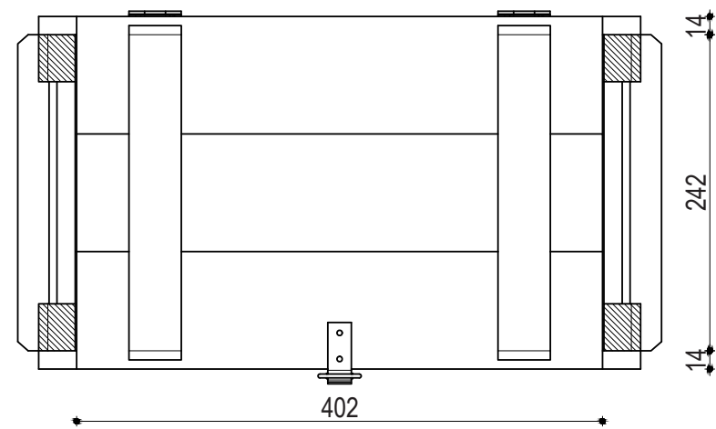
BOVENAANZICHT
