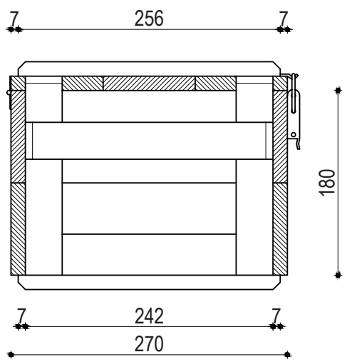
ZIJAANZICHT
