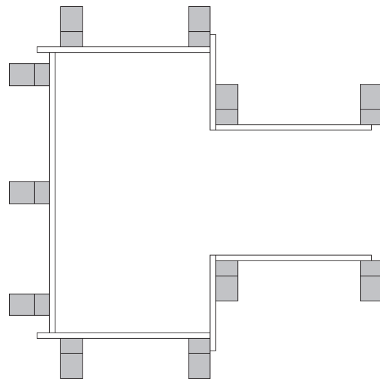
BOVENAANZICHT BEKISTING
