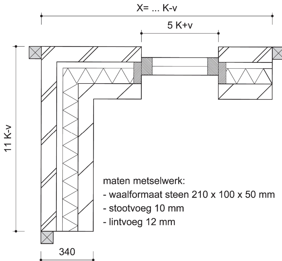
BOVENAANZICHT SPOUWMUUR
