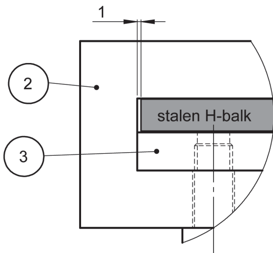
DETAIL A schaal 1:1
