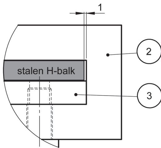
DETAIL B schaal 1:1
