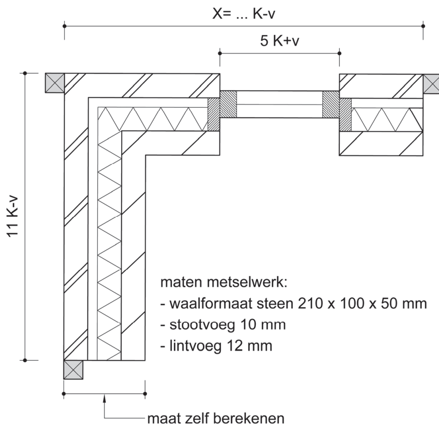
BOVENAANZICHT SPOUWMUUR
