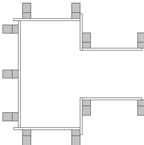
BOVENAANZICHT BEKISTING
