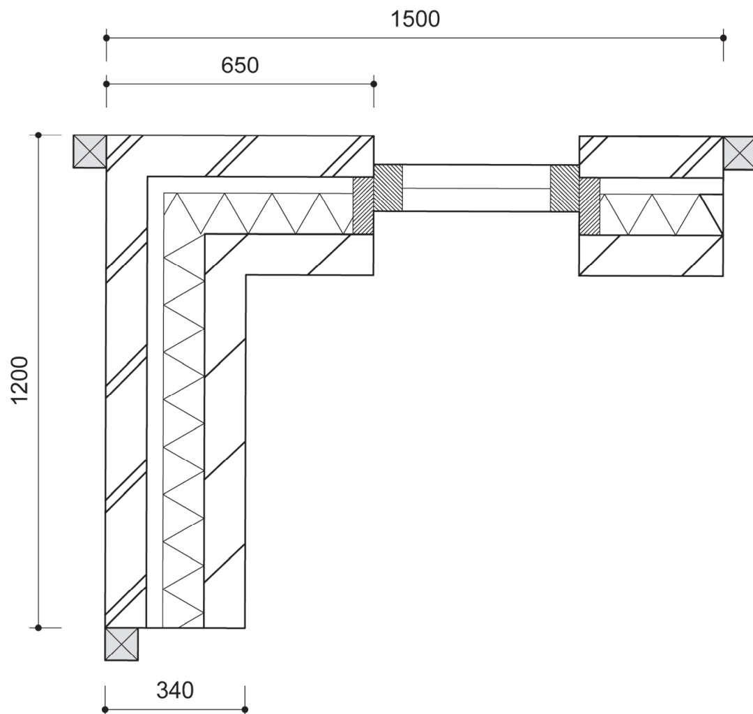
BOVENAANZICHT SPOUWMUUR
